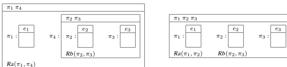
Figure 3: SDRS correspondant à (A) et (B)
