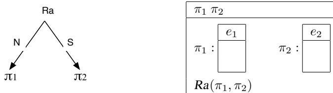
Figure 1: LODAG et SDRS pour SI\ Conj_a\ S2
