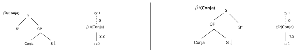
Figure 5: Arbres auxiliaires et arbres de dérivation pour les subordinées postposées et préposées
